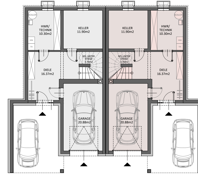
TOP 1 TOP 2 ✓ Kellergeschoß Top 1 59,45 m 2 | Top 2 59,45 m 2 (je 3,75 m 2 unter Stiege)
